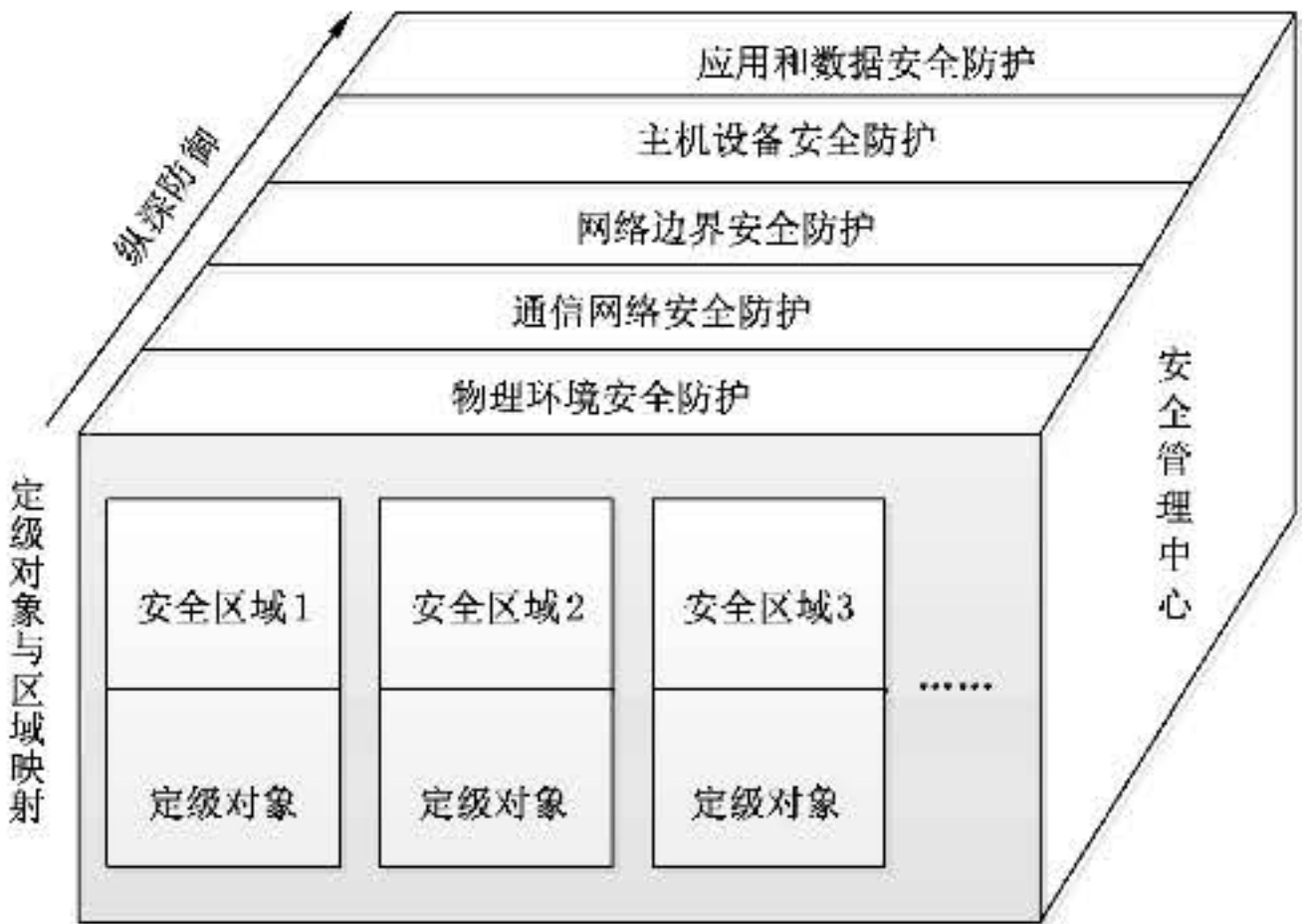
图 4 等级保护对象的安全技术体系架构
